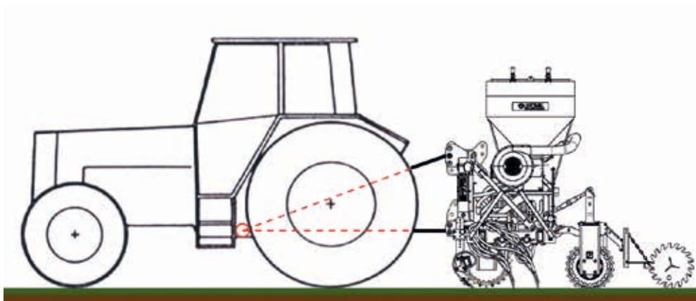
Attelage arrière en position de travail
