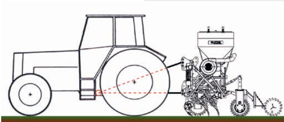
Heckanbau in Arbeitsposition
