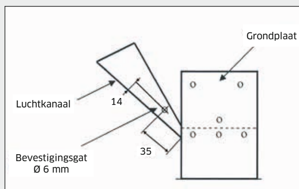
Montage van de hectareteller
